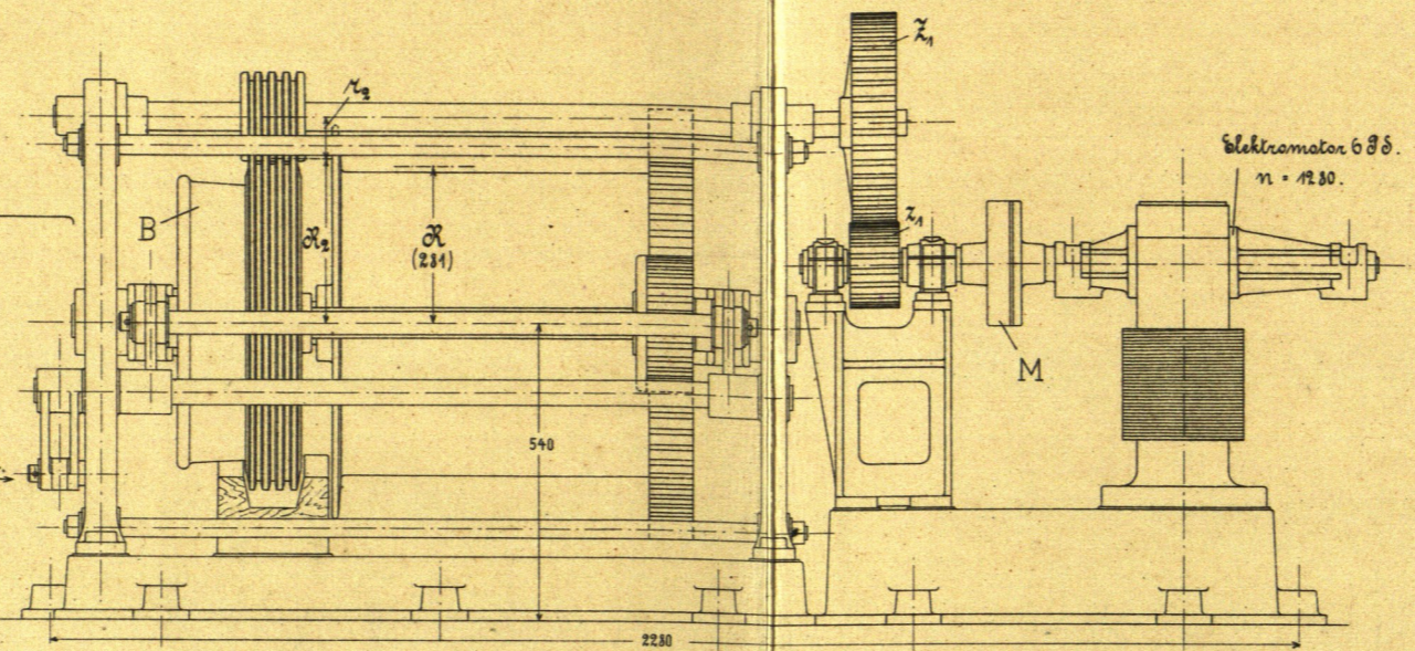
Fig. 2. 1/5. Klassische Maschinenbau Soc. Srafenstaden.
