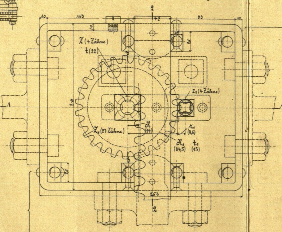
Fig. 2. 1/5. Klassische Maschinenbau Soc. Srafenstaden.
