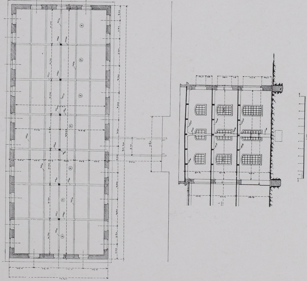
Sämtliche Decken, Säulen und Dächer in armiertem Beton System Ast & Co.
