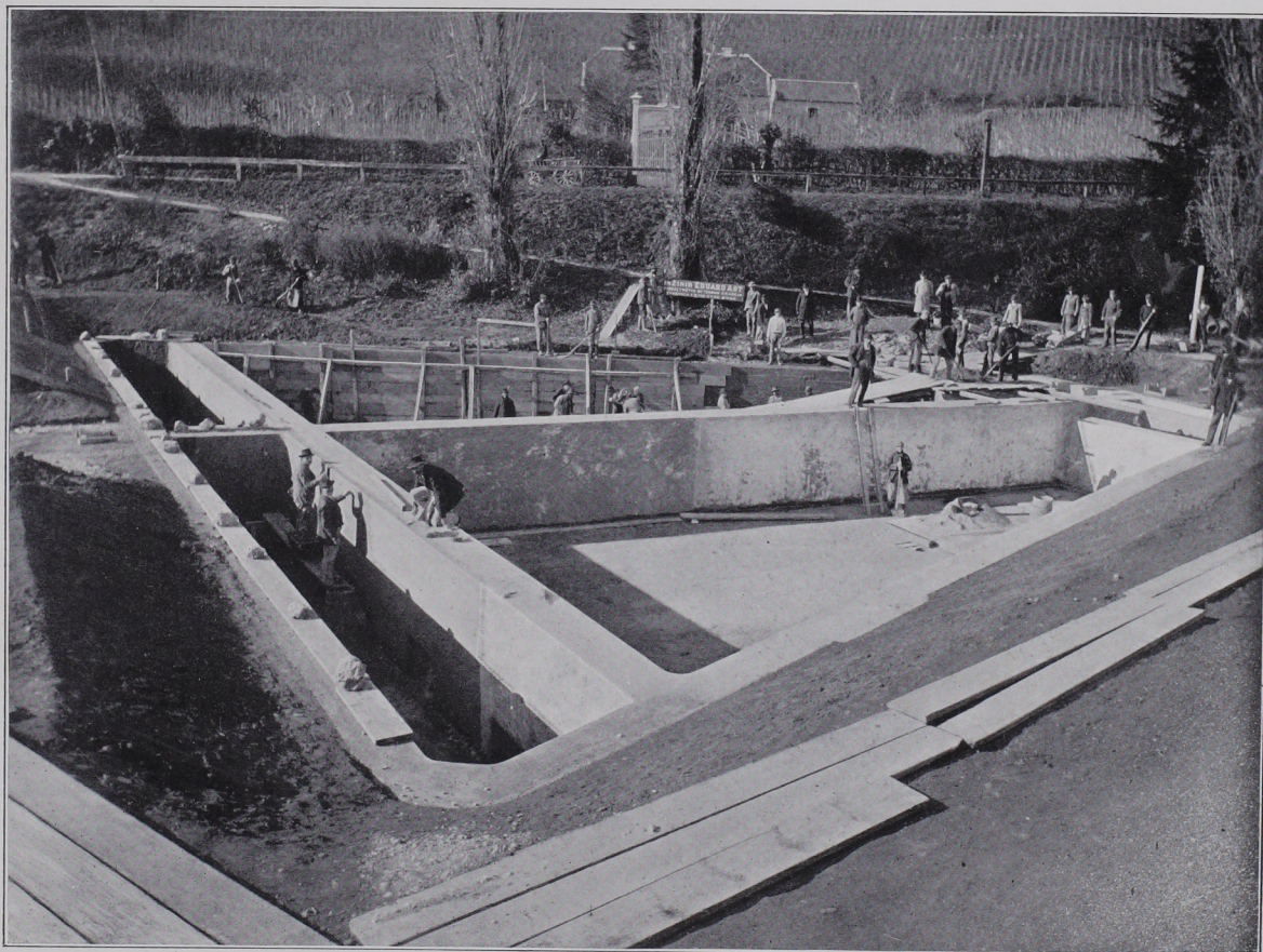
Hergestellt in Portlandzement-Stampfbeton mit wasserdichtem Putz. Ausgeführt im Jahre 1898.
