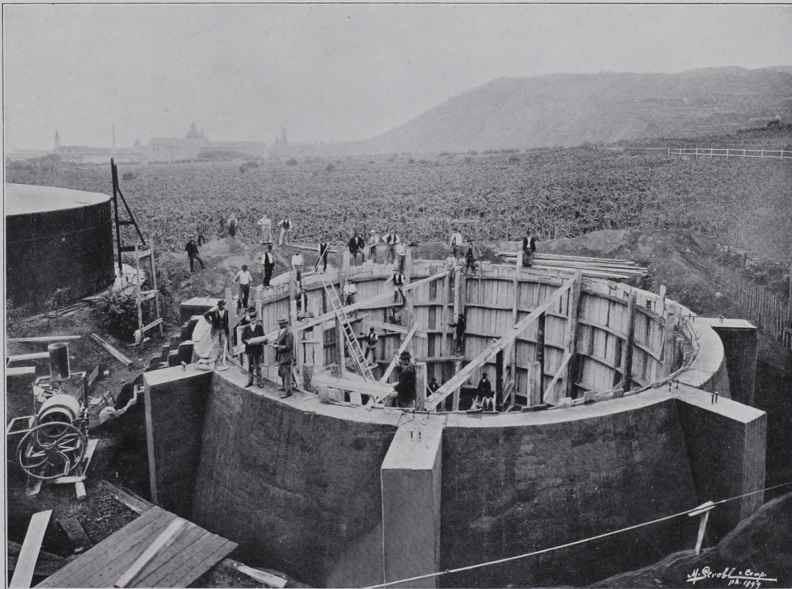
Ausgeführt im Herbst 1899. Lichter Durchmesser 14,5 m, lichte Höhe 6,4 m.
