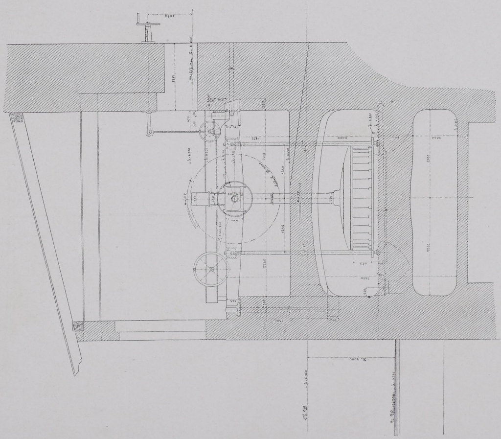
Turbinen-Einbau und Unterwassergraben in Portlandzement-Stampfbeton.
