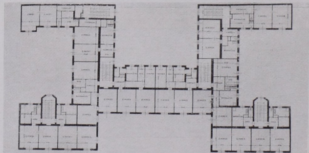
Stockwerksplan
