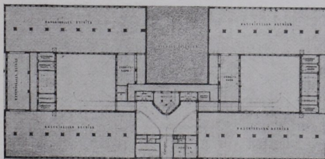
Erdgeschoß
