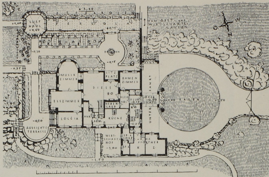
Plan vom Erdgeschoß und Garten
