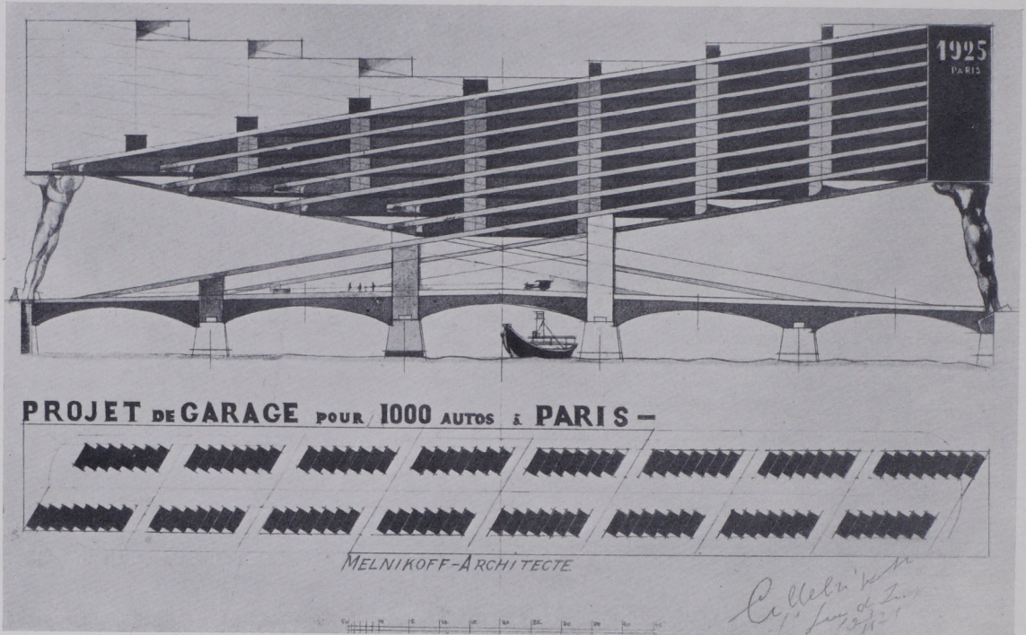
Abb. 102. K. Mjelnikow. Entwurf einer Großgarage für Paris.
