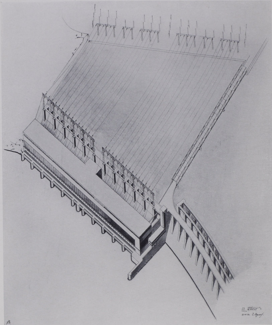
Abb. 89. Kraftwerk Dnjeprostroi. Entwurf: Architektur-Abteilung der Bauleitung. Arch. W. Wjesnin. Mitarbeiter: N. Kolli, G. Orlow, S. Andreewski.
