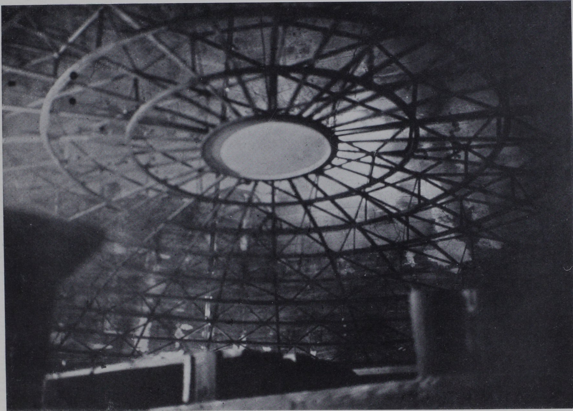
Abb. 86. Montage der Kuppel im Planetarium, Moskau.
