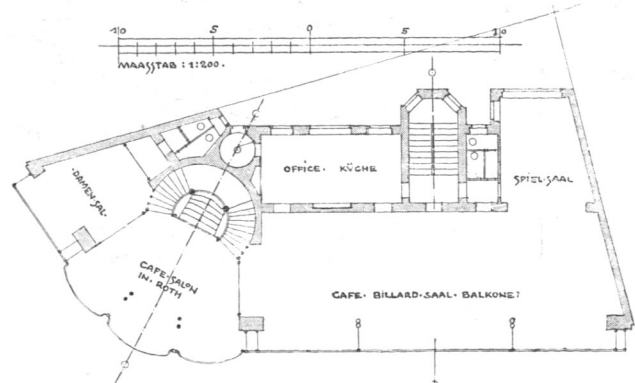
GRUNDRISS ERSTER STÖCK •
