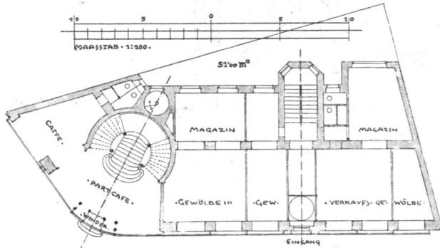
• GRUNDRISS PARTERRE •
