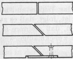
Abb. 961 bis 963. Kolbenringeschlösser.
