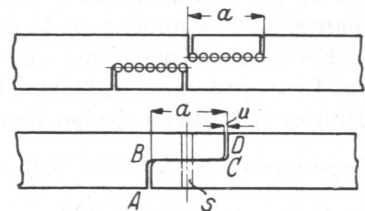
Abb. 958. Ausbohren des Kolbenringschlösses.
