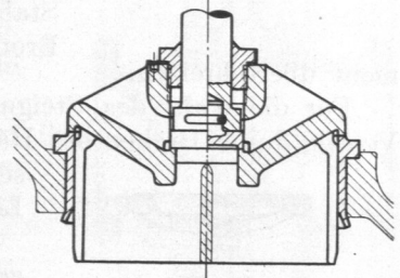
Abb. 751a. Voröffnungsventil.
