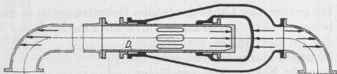
Abb. 732. Entlasteter Stopfbuchsausgleicher.
