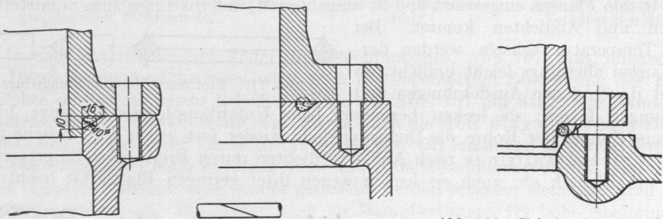
Abb. 714 und 715. Gummischnurdichtungen.
