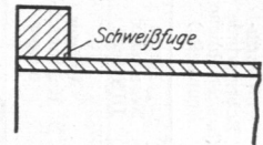
Abb. 672. Bordring aufgeschweißt.
