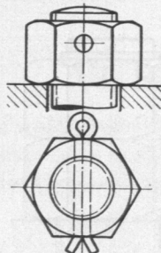
Abb. 396. Splint- sicherung.
