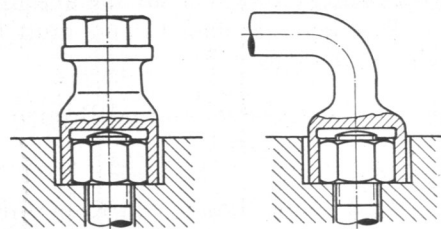
Abb. 361 und 362. Steckschlüssel.
