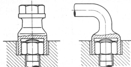
Abb. 361 und 362. Steckschlüssel.
