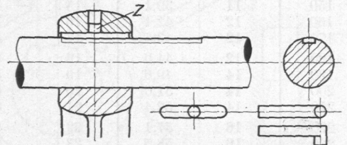
Abb. 313. In einer Nut gleitende Feder.
