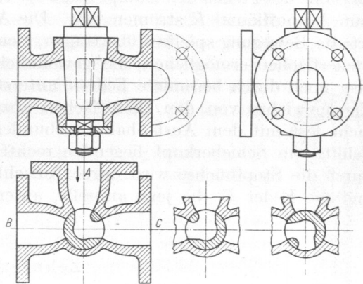
Abb. 874. Dreiweghahn.
