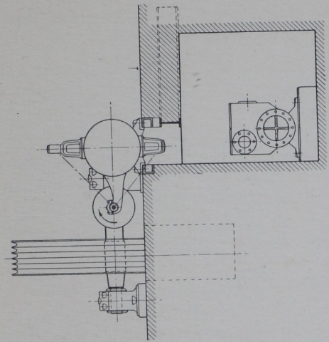
Dispositions - Skizze einer liegenden Einzylinder - Maschine mit Kondensation.
