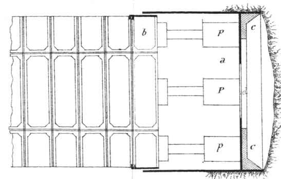
Cassone pel sifone Clichy - Cbsnières sotto la Senna
