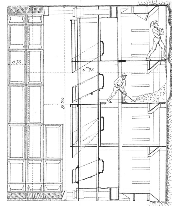
Cassone per la galleria Blackwal sotto il Tamigi
