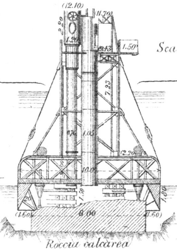
Esecuzione della muratura
