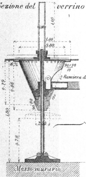
Scala di 1:40
