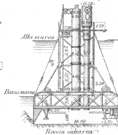
Spianamento del fondo
