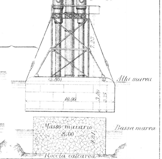
Cassone in galleggiamento
