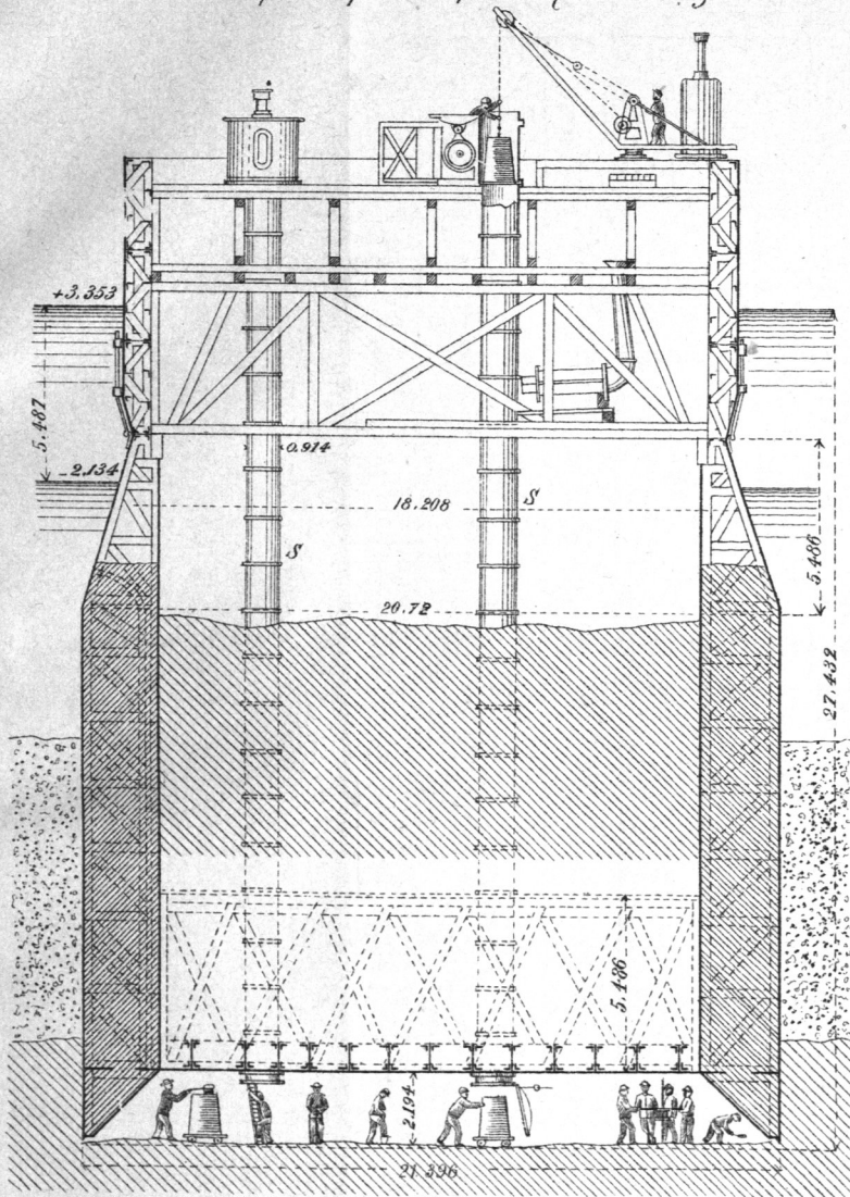
Fig. 32 Ponte sul golfo di Forth Cassone per le pile del pilone Queensferry
