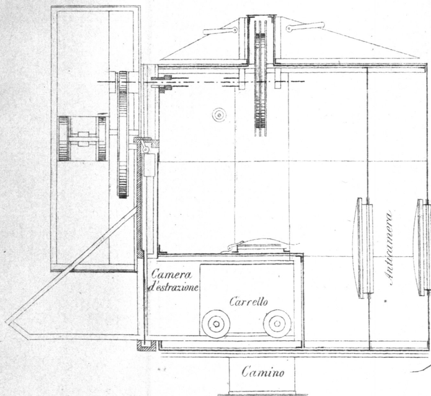
Ponte a Mezzanacorti Particolari della camera d'equilibrio
