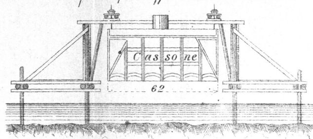
Castello fisso per l'affondamento del cassone
