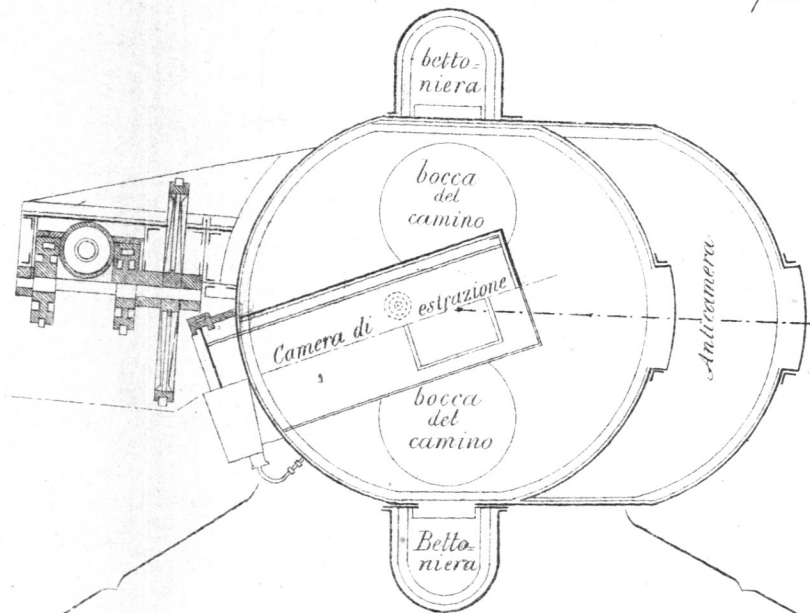
Ponte a Mezzanacorti Particolari della camera d'equilibrio
