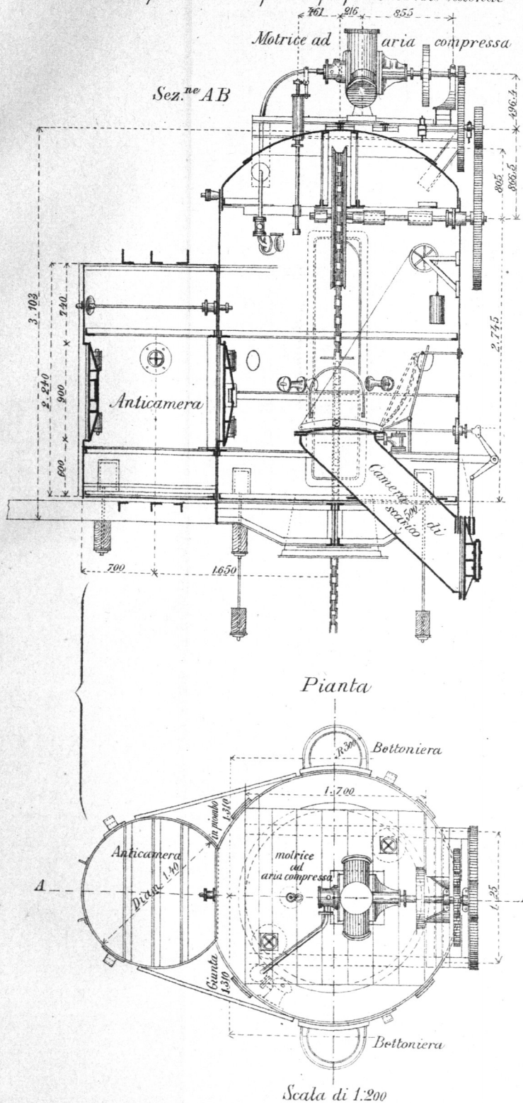
Fig. 18. Particolari della camera d'equilibrio-con anticamera, camera d'estrazione e betoniere
