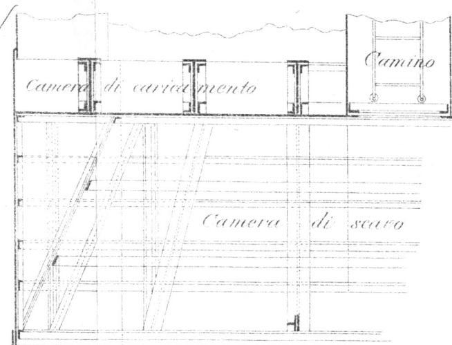
Scala di 1:50
