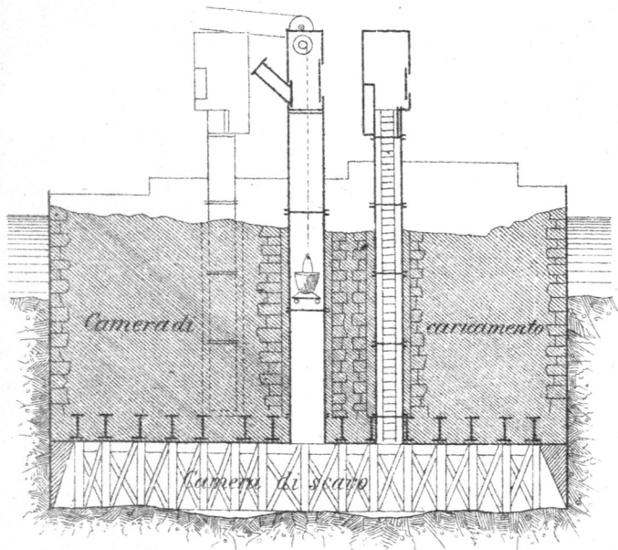
Scala 1:200
