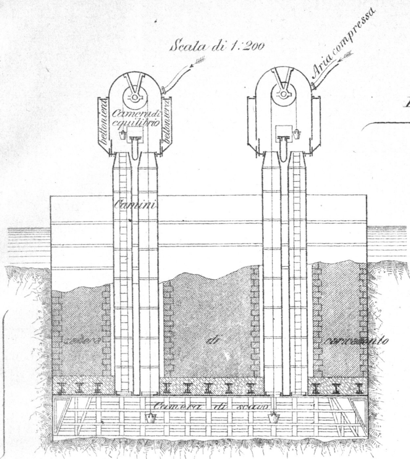
Pontone Garibaldi a Roma
