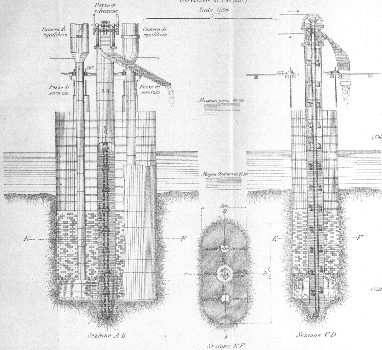
Fig. 8 Ponte a Piacenza (Fondazione di una pila) Scala 1/200
