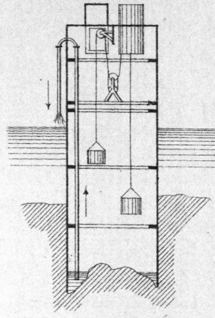
Fig. 2. Metodo Hughes (Ponte Medway)
