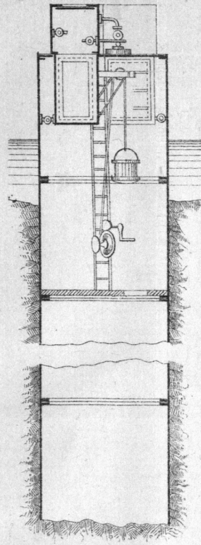
Fig. 5. Metodo Fleur St Denis (Ponte Kehl)
