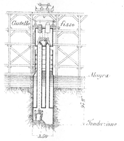
Fig. 4. Metodo Cézanne (Ponte Kowno)
