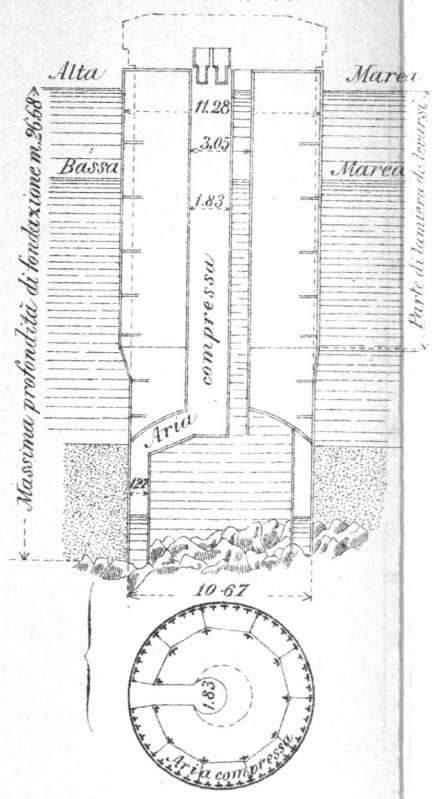
Fig. 7 Ponte Argentueil
