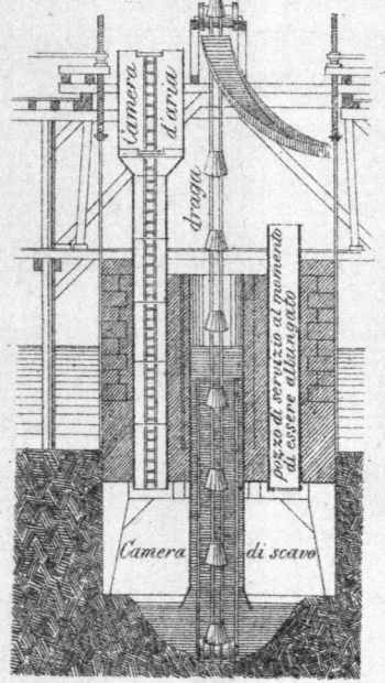
Fig. 5. Metodo Fleur St Denis (Ponte Kehl)
