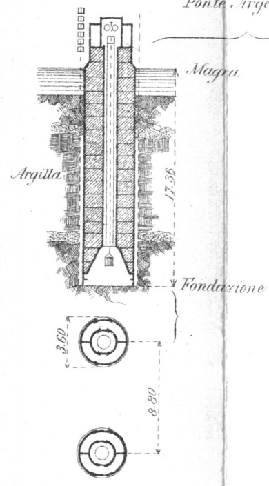
Fig. 7 Ponte Argentueil
