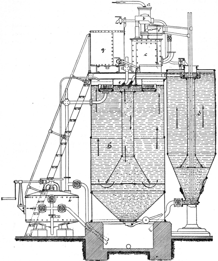
Fig. 38. Apparat zur Reinigung von Kesselspeisewasser Breda II.
