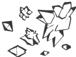
Fig. 14 Sandoptal-Kupfer-Ammoniak.
