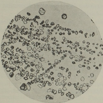
Fig. 2. Sublimat von Vanillin.
