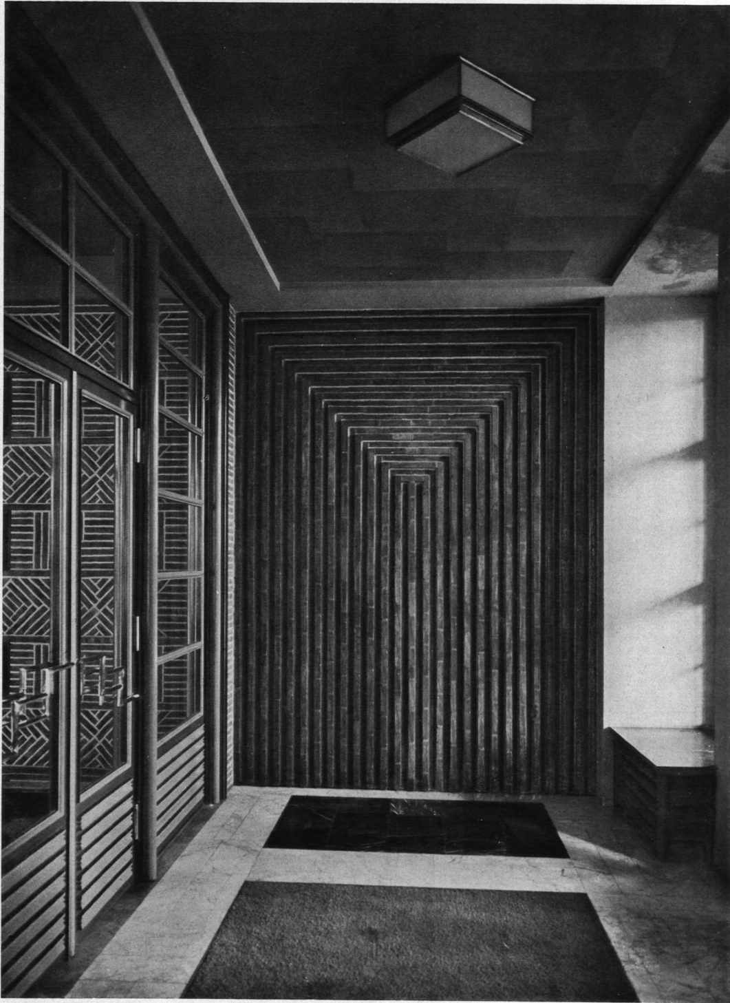
Büro- und Wohlfahrtsgebäude. Windfang
