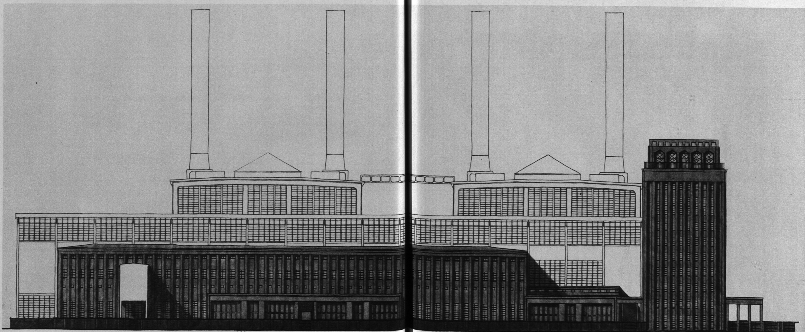
Großkraftwerk Klingenberg — 30000 Volt-Schaltheis (oben) — Maschinenhausvorbauten und Bürohaus
