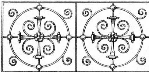
Schmiedeeiserne Füllungsgeländer.
