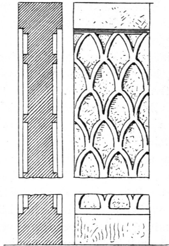
Von der Stoa des Königs Attalos II. zu Athen 17) .
