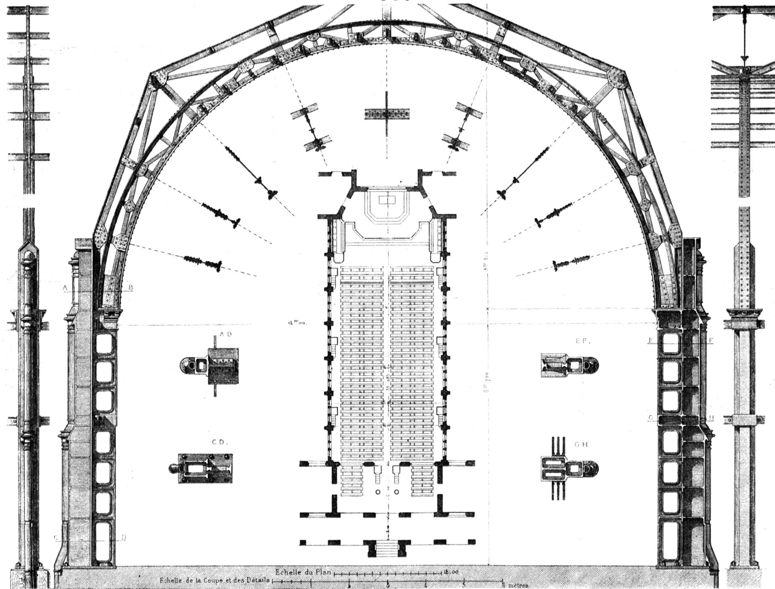
Capelle der Maison de force et de correction zu Rennes. — Arch.: A. Normand 536).
