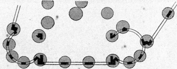
Von den magasins du Printemps in Paris. Theil des Fundament-Planes 223) . — 1/500 n. Gr.
