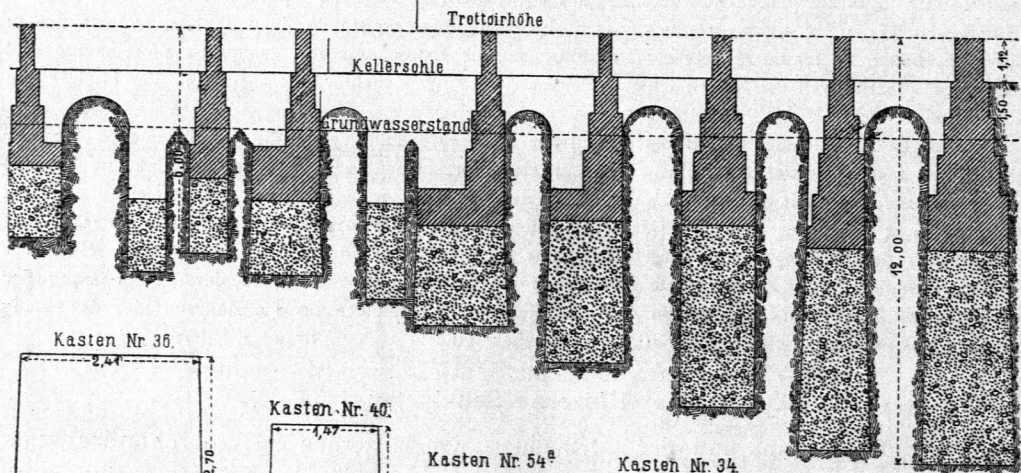
Fig. 738. Schnitt durch die Fundamente nach M N.
