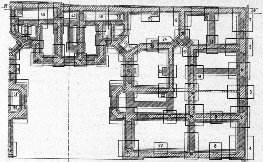
Fig. 737. Grundriß des Erdgeschosses und Fundament-Plan.
