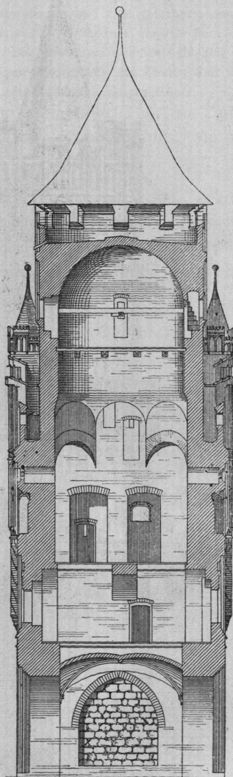
Schnitt.
