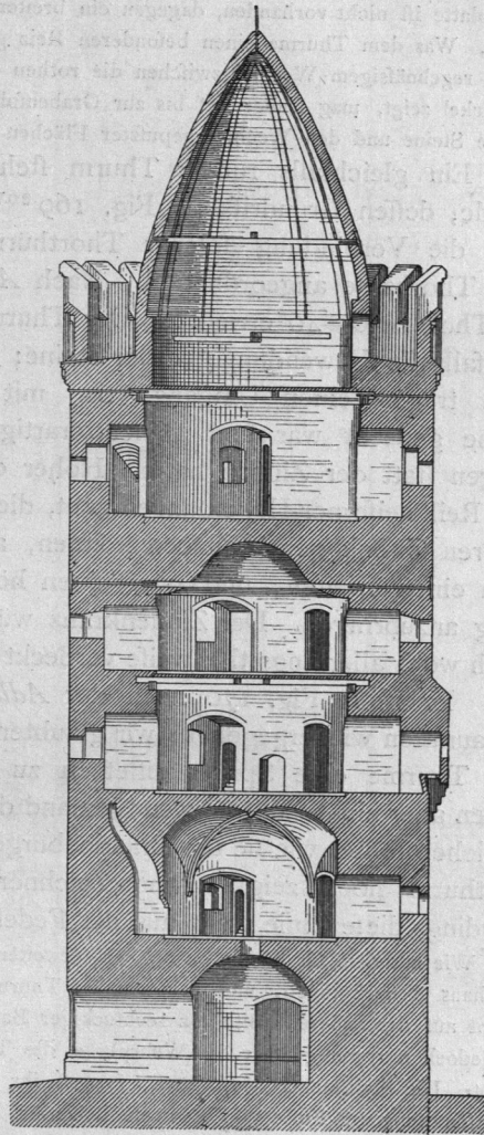
Schnitt.
