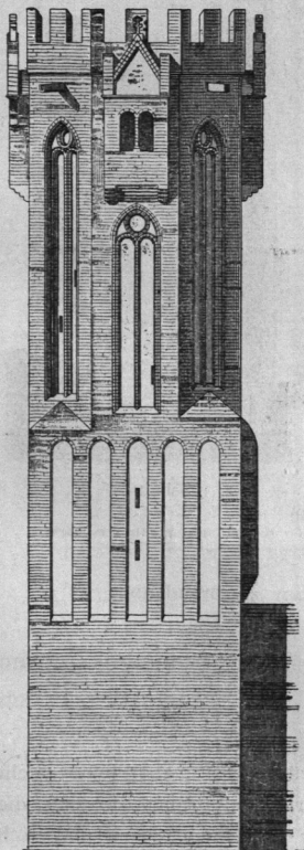
Thurm am Hühnerdorfer Thor zu Tangermünde 203) . 1/250 n. Gr.
