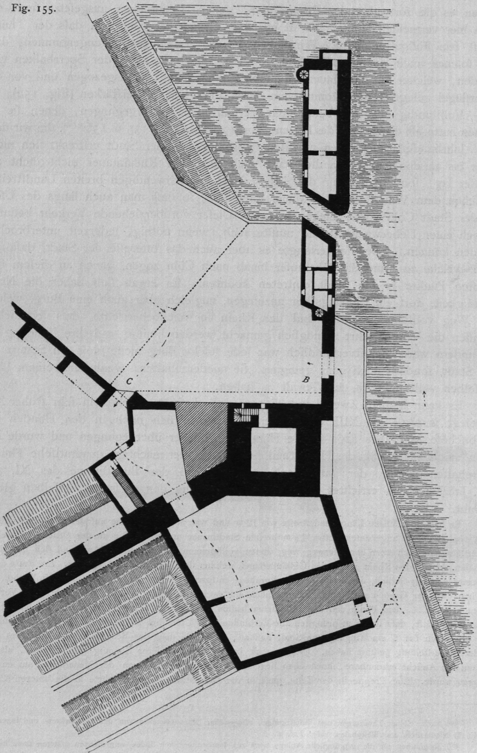
1:500 10 9 8 7 6 5 4 3 2 1 0 5 10 15 20 m Bayen-Thor zu Cöln mit Vorwerken 200 ).
