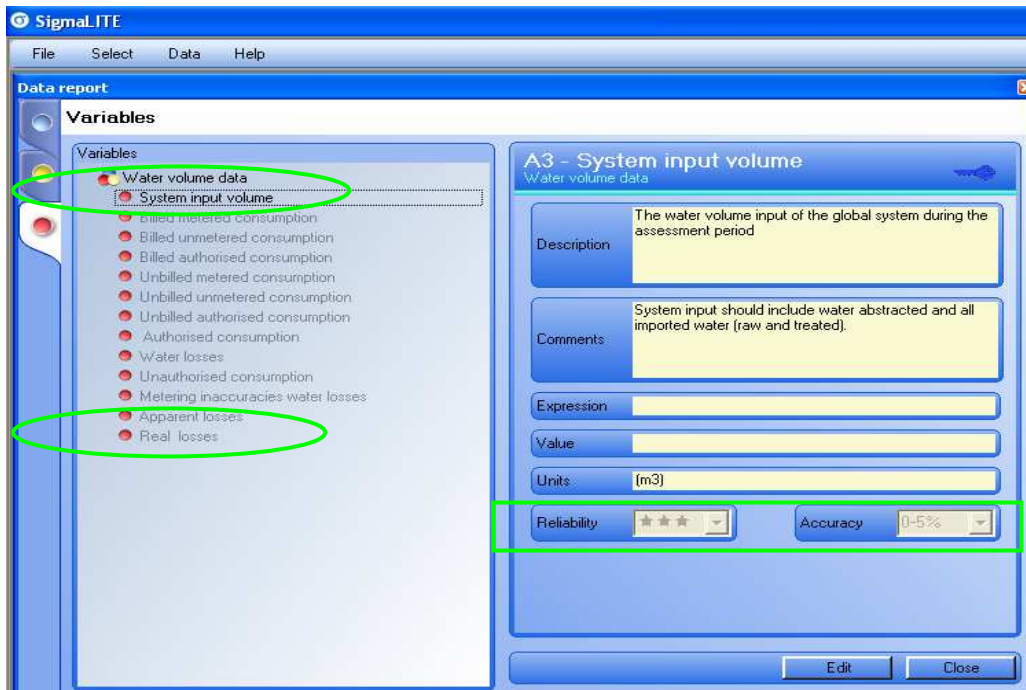
Abbildung: 22: Sigma Lite 2.0 Variables- Water volume data – „System input volume“
