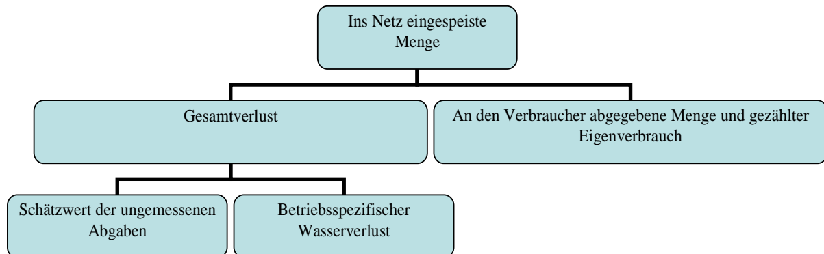
Abbildung 49: Datenelemente zur Erstellung einer Wasserbilanz nach der ÖVGW-Richtlinie W 63
