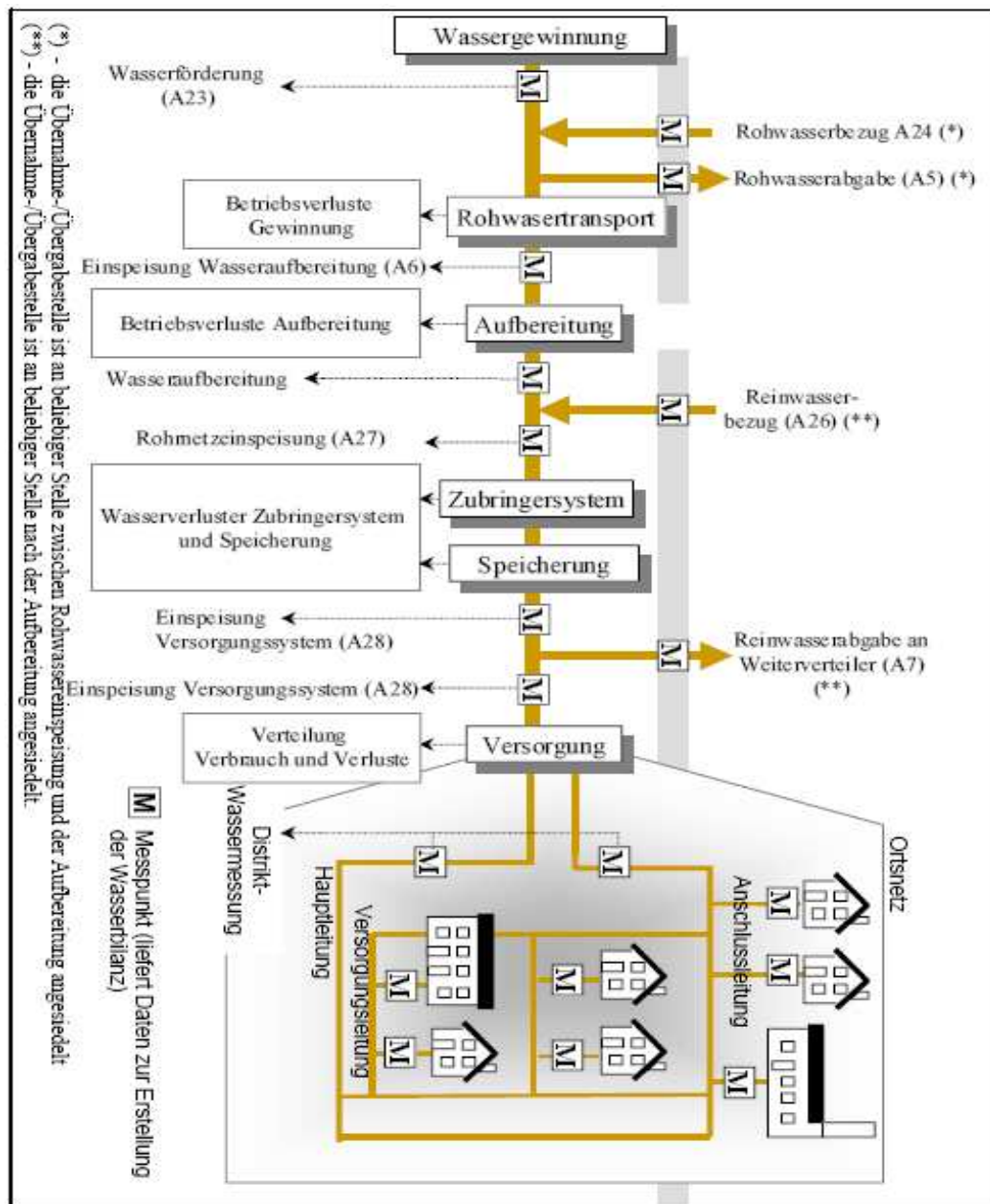
Abbildung 51: Grundschema einer Wasserbilanz nach Alegre et al. 2000
