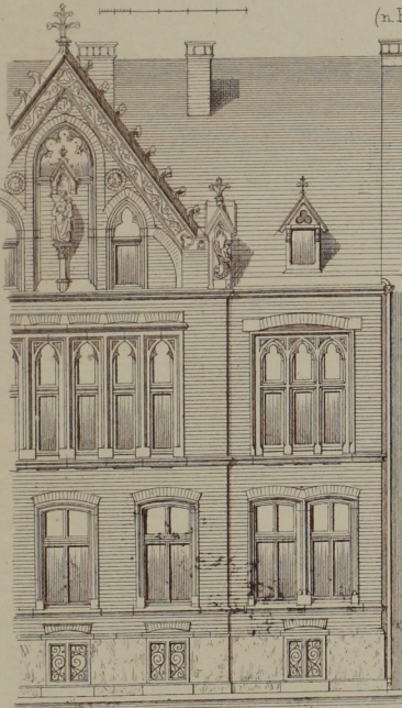
Wohnhaus in Aachen. (n. V. Statz.) (M. f. H. 1874)
