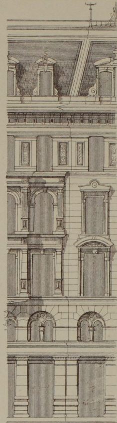
Geschäfts- & Wohnhaus - Berlin. (n. Bodenwoldt) (M.H. 1874)
