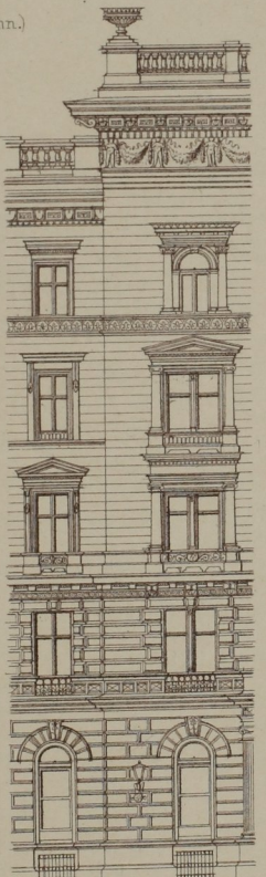
Fig. 1496. Grand Hotel -Wien. (n. K. Titz) (A. B. 1871)
