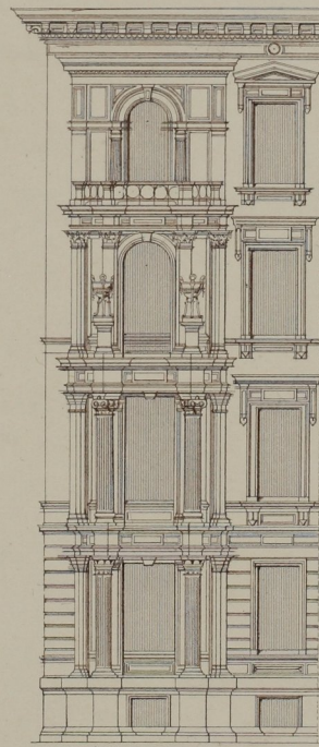
Fig. 1471. Miethaus-Berlin n. O. Titz. (M.f. H. 1874)
