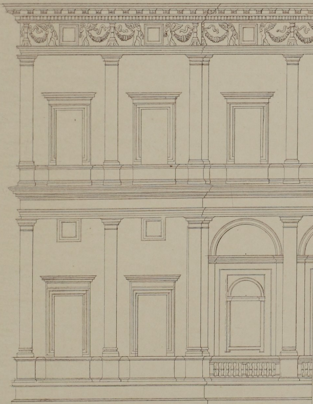
Fig. 1427. Pal. Comunale zu Brescia (it. Ren.) (n. Nohl)
