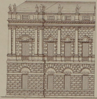
Pal. Tiepolo zu Vicenza. Theil der Façade (it. Ren.) (n. Burckhardt)
